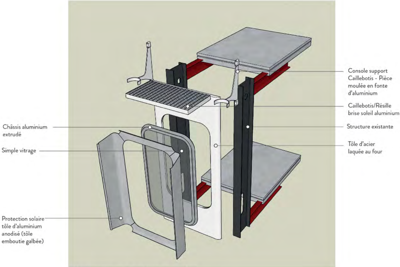
ETAT EXISTANT D'UNE TRAME DE FACADE
