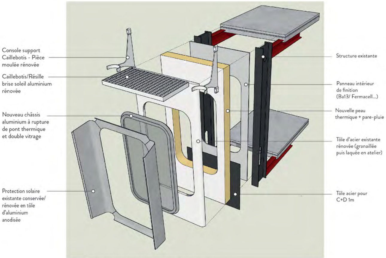
PRINCIPE PROJETE D'UNE TRAME DE FACADE
