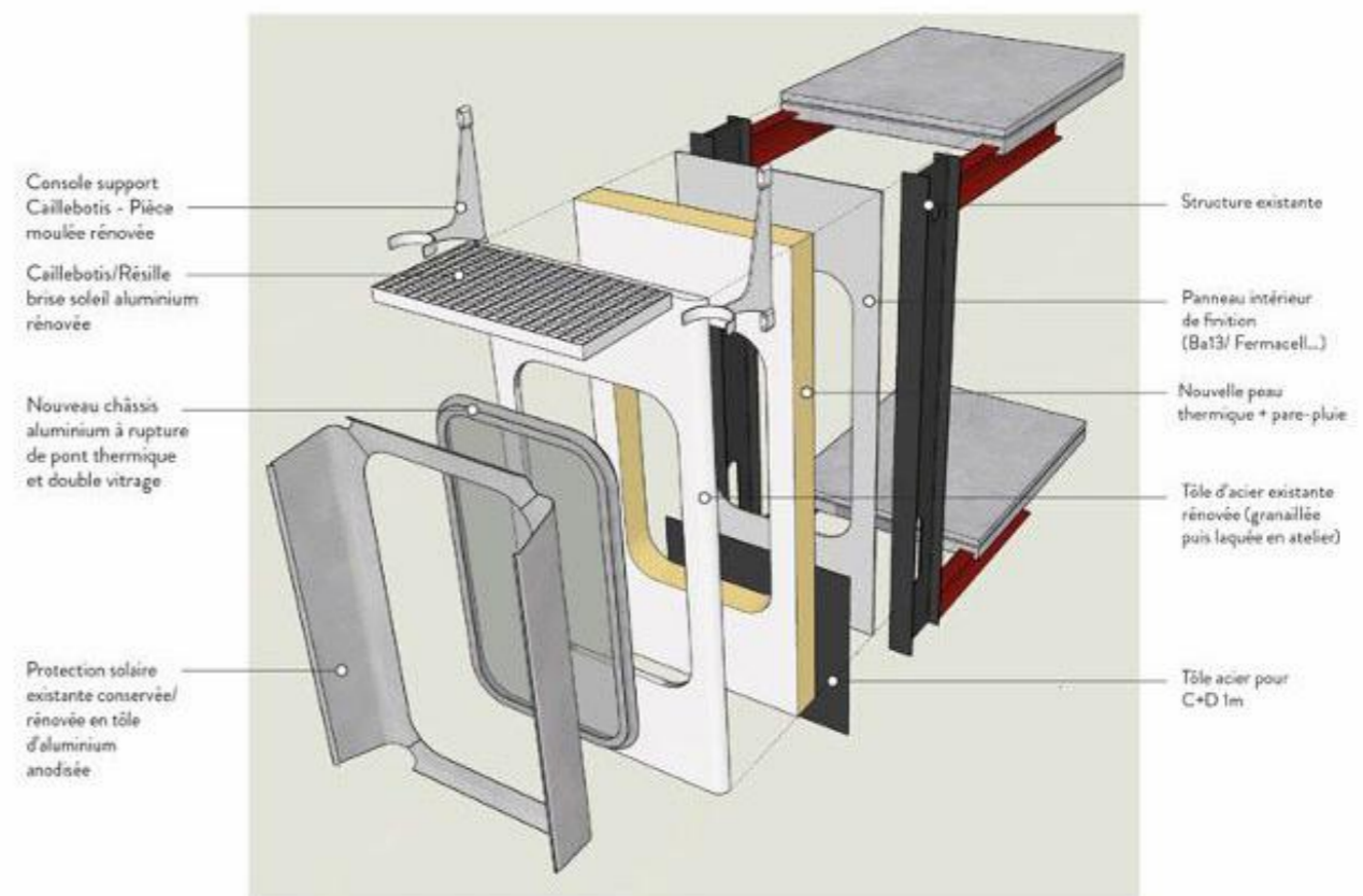
PRINCIPE PROJETE D'UNE TRAME DE FACADE
