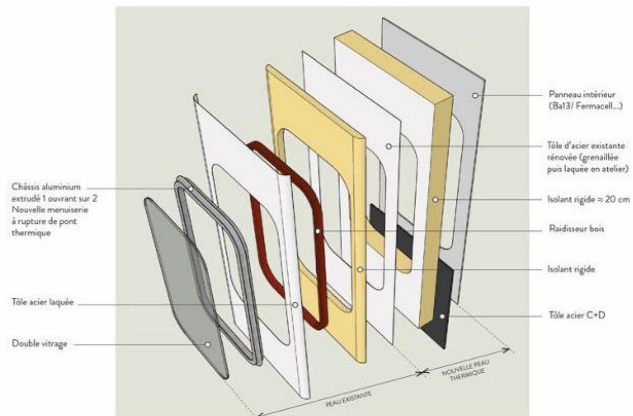
PRINCIPE PROJETE D'UN PANNEAU DE FACADE
